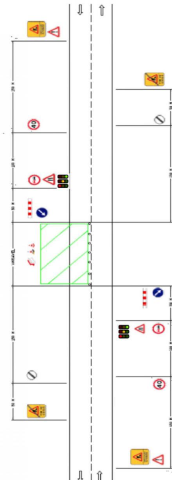
ESQUEMA TIPO 2 – SINALIZAÇÃO DAS VIAS PÚBLICAS FORA DAS LOCALIDADES COM A UTILIZAÇÃO DE SEMÁFOROS
