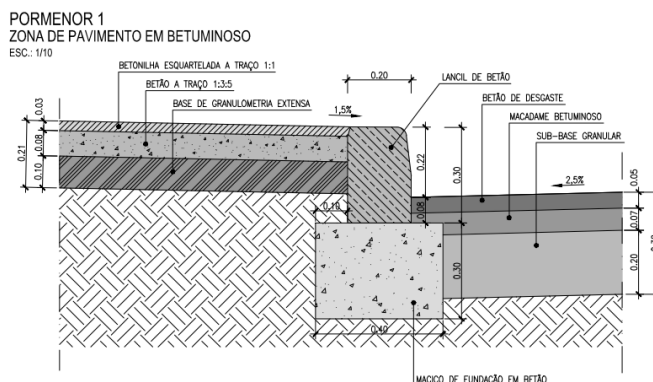
Fig. 3 – Pormenor do pavimento em betão betuminoso e passeio
