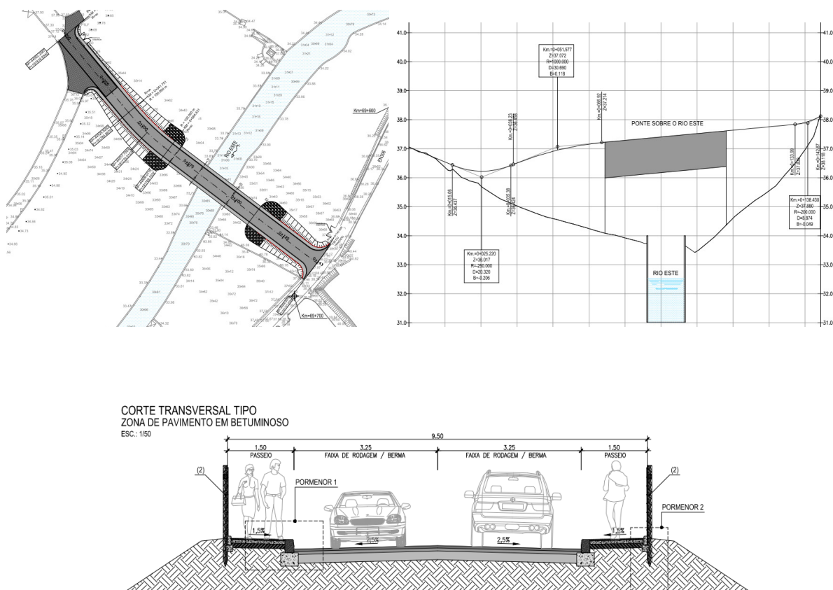
Fig. 1 - Perfil Transversal Tipo
