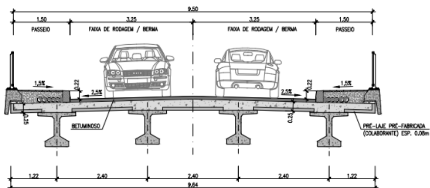
CORTE TRANSVERSAL (ZONA CORRENTE) ESC.: 1/50
